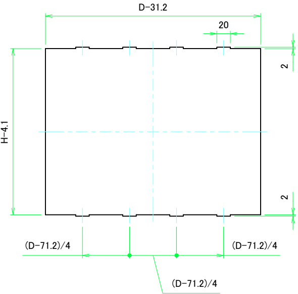
Dパネル1表面 / D Panel 1 Frontside
