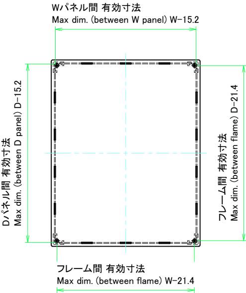
下カバー / Bottom cover
