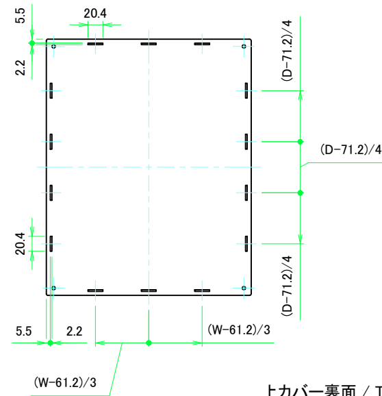
上カバー裏面 / Top cover Backside
